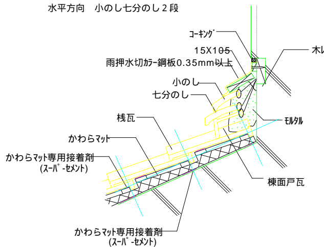
壁ぎわRC造・かわらマット工法 水平方向 小のし七分のし 2段
