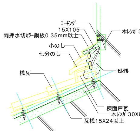
壁ぎわRC造・口式縦棧工法 水平方向 小のし七分のし 2段
