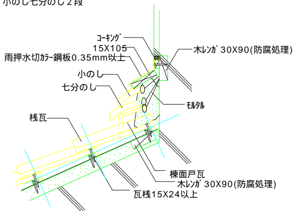
壁ぎわRC造・P-ライト珧外工法 水平方向 小のし七分のし 2段
