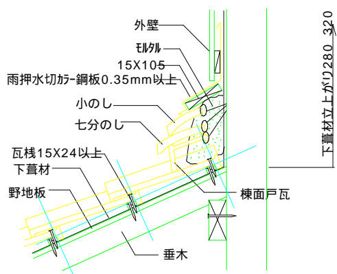
壁ぎわ木造・在来工法 水平方向 小のし七分のし 2段
