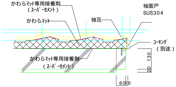
右けらばRC造・かわらマット工法
