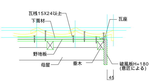
右けらば木造・木地仕上げの破風
